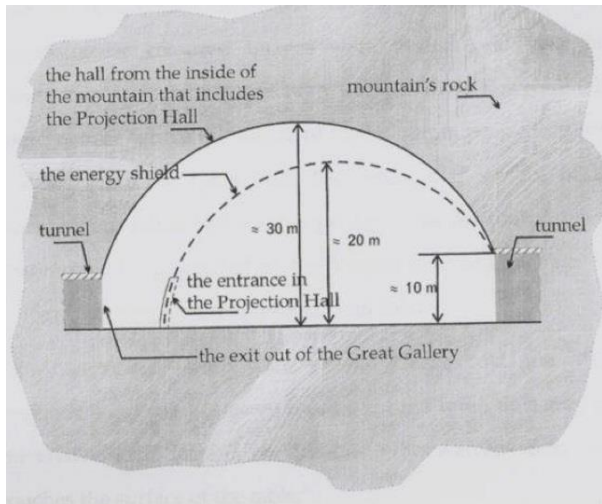
Schema projekčního sálu z boku ve skalách pohoří Bucegi - Rumunsko nebeska-univerzita.cz
